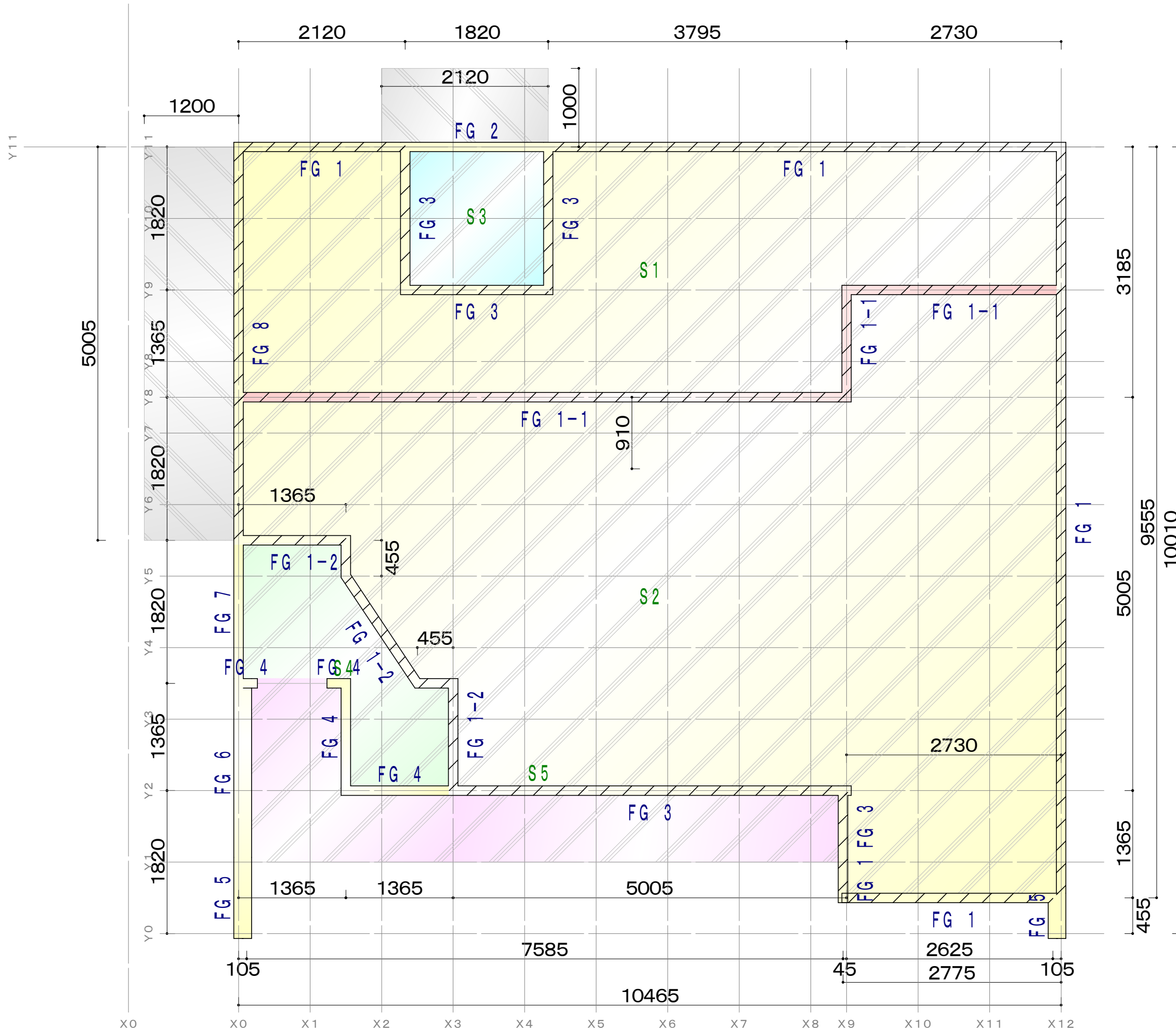
1階：基礎伏図
